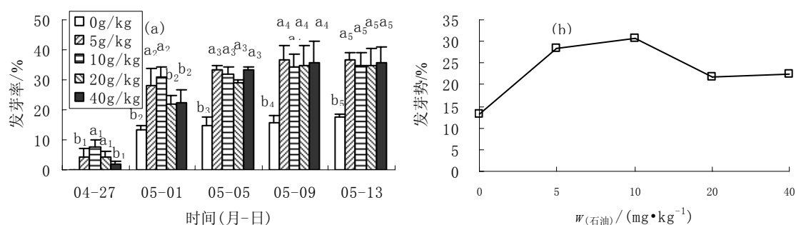
图3 不同质量分数石油烃对碱蓬发芽率(a)和发芽势(b)的影响
